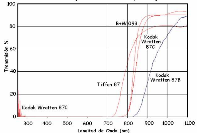
Filtros Infrarrojos mas Comerciales que se Ajustan
