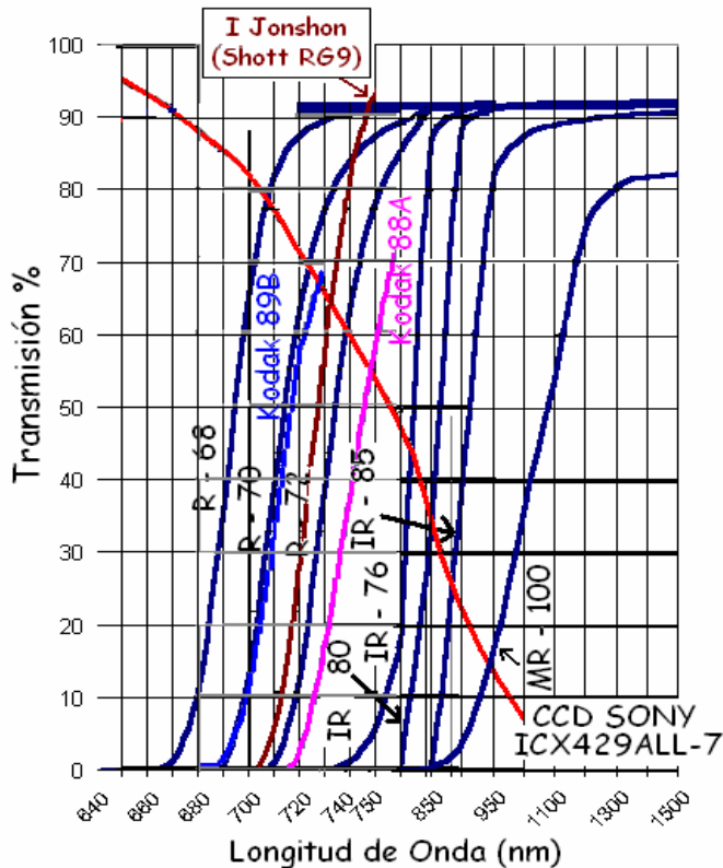
Filtros Rojos e Infrarrojos vs CCD y Filtro I Jonshon (Shott)
