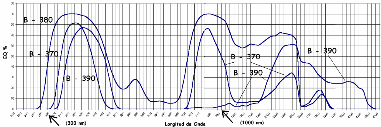
Filtros Hoya Azules B - 370, 380 y 390
